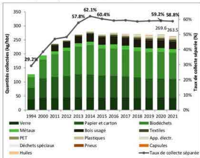
Figure 3 : Détail de l'évolution des fractions recyclables, kg par habitant
